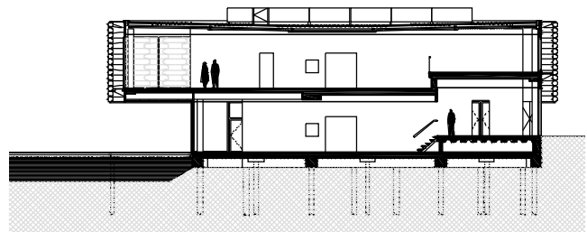
langsdoorsnede
