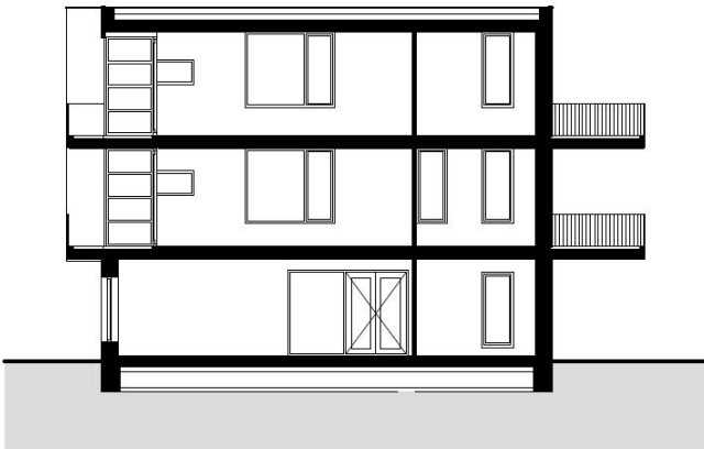
dwarsdoorsnede
