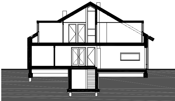
dwarsdoorsnede
