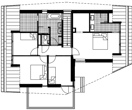
verdieping
